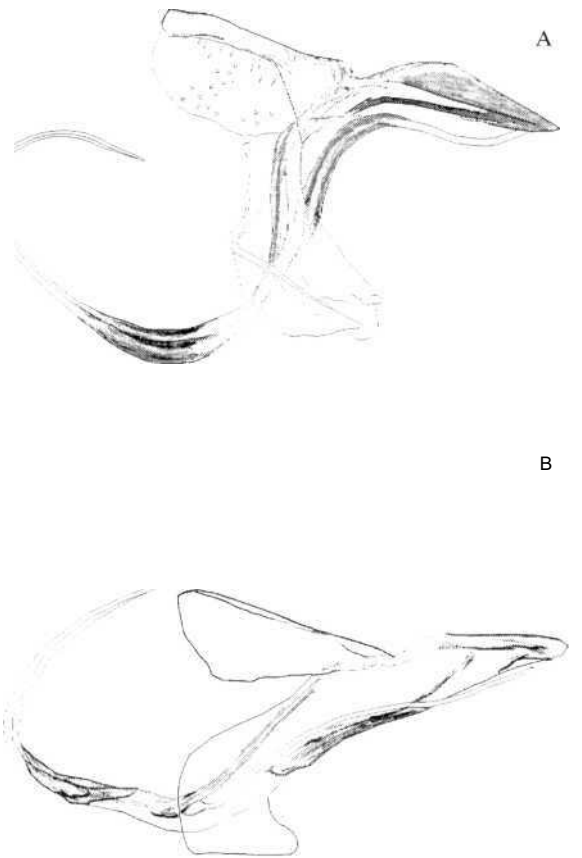
Fig. 3. Ophiomyia bohémica (A) and O. heracleivora (B) male genitalia. Aedeagus 3 pav. Ophiomyia bohémica (A) ir O. heracleivora (B) patinų genitalijos. Aedeagus
